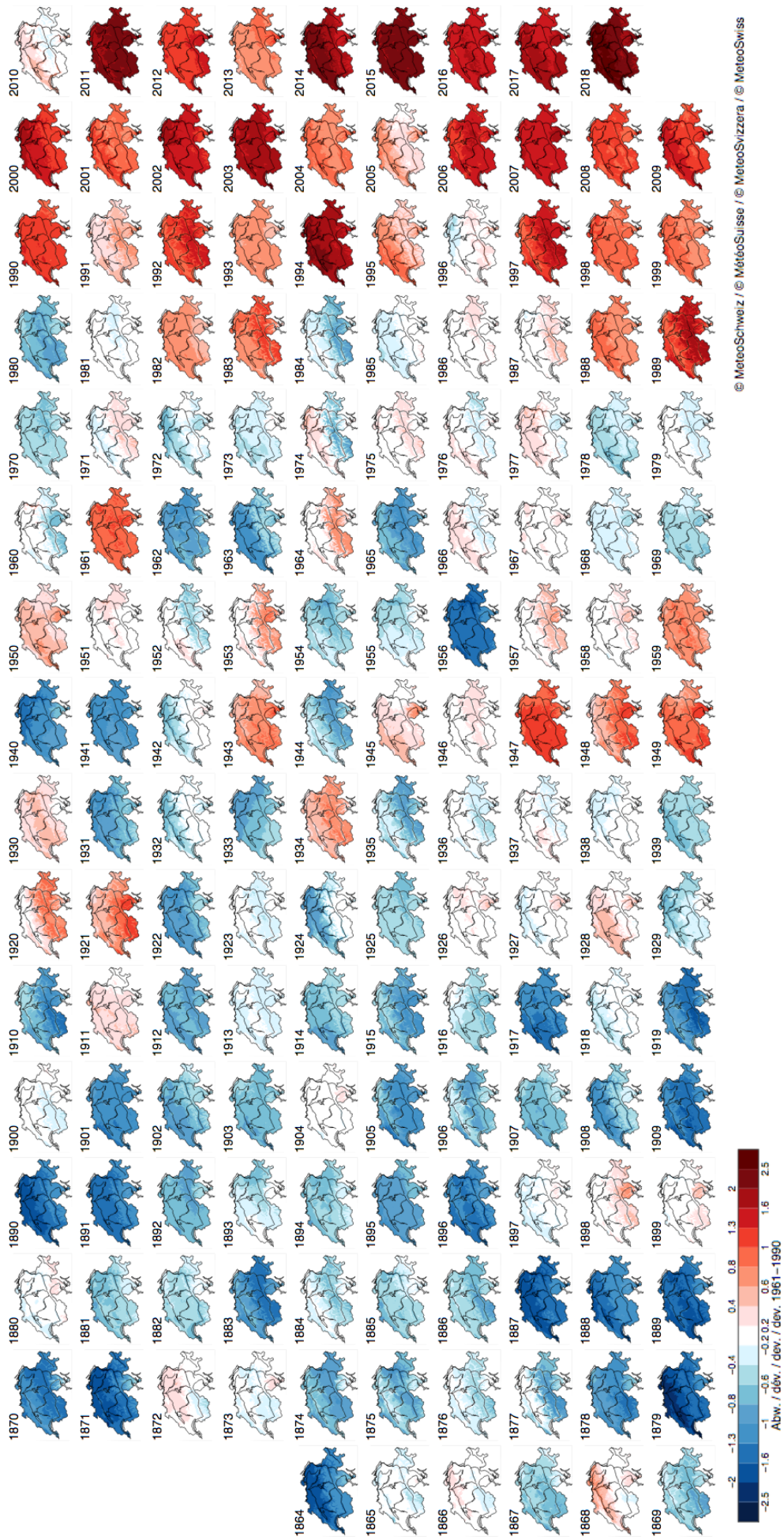
Die Grafik zeigt die Abweichung der Jahrestemperatur im Vergleich zum Durchschnitt von 1961-1990. Alle Jahre unter dem Durchschnitt sind blau eingefärbt, alle Jahre über dem Durchschnitt sind rot. (Quelle: meteoschweiz.ch)
