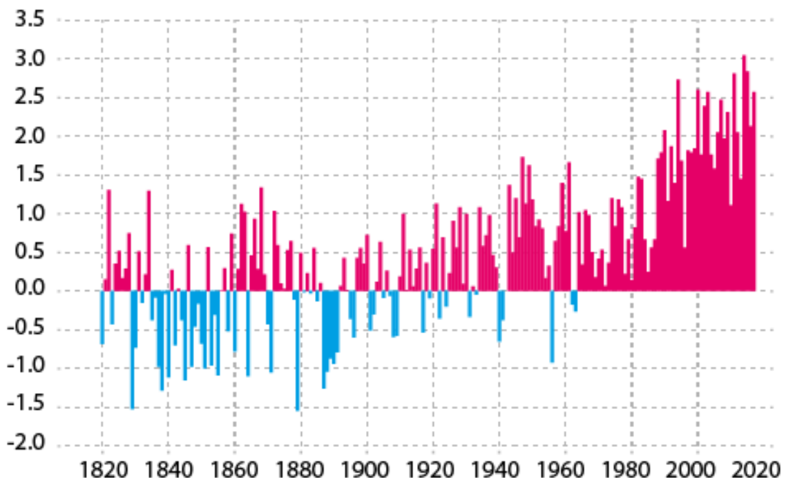
Abweichung Jahrestemperatur Basel in ^{\circ}\text{C}
